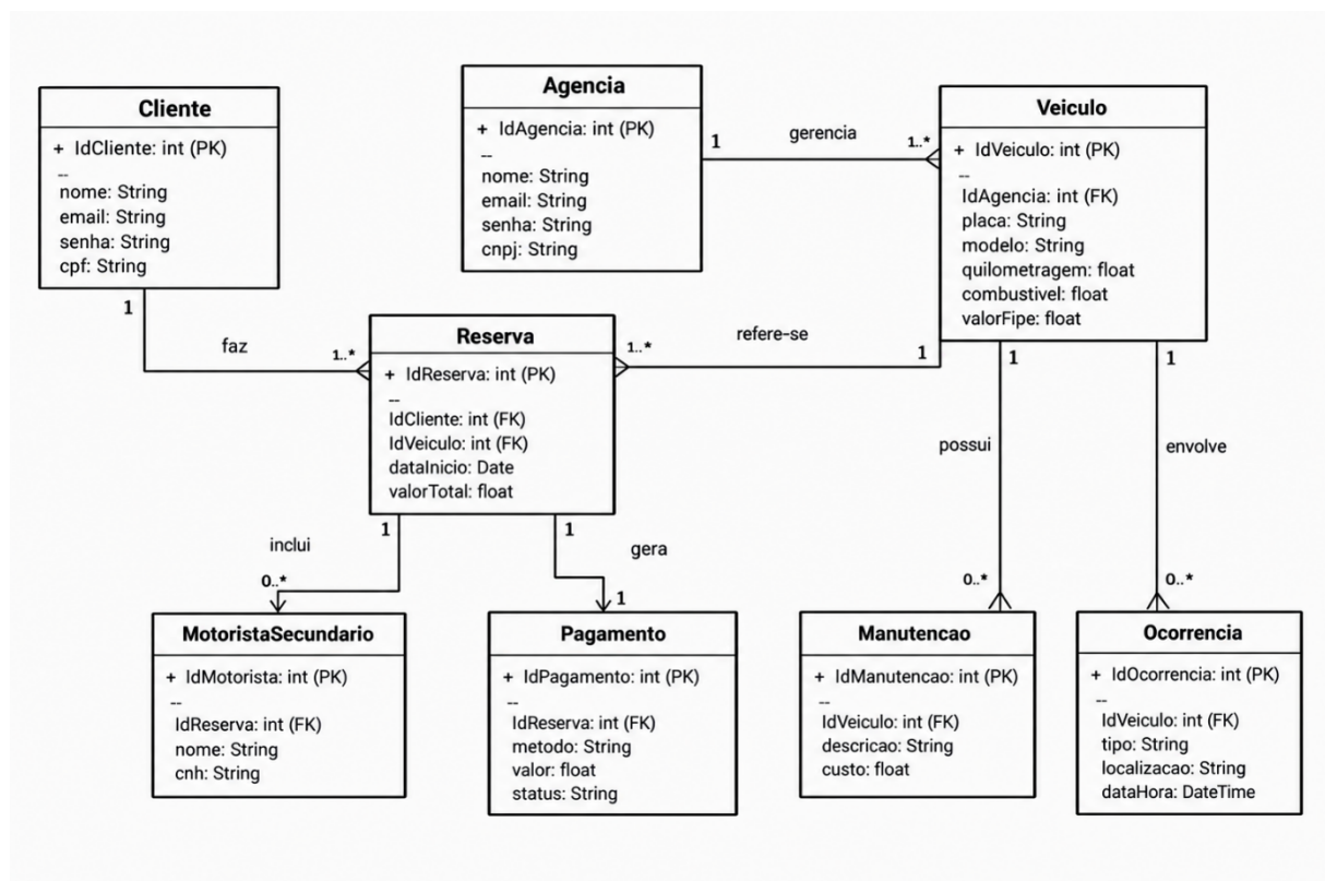
Figura 5.3: Diagrama Entidade-Relacionamento
