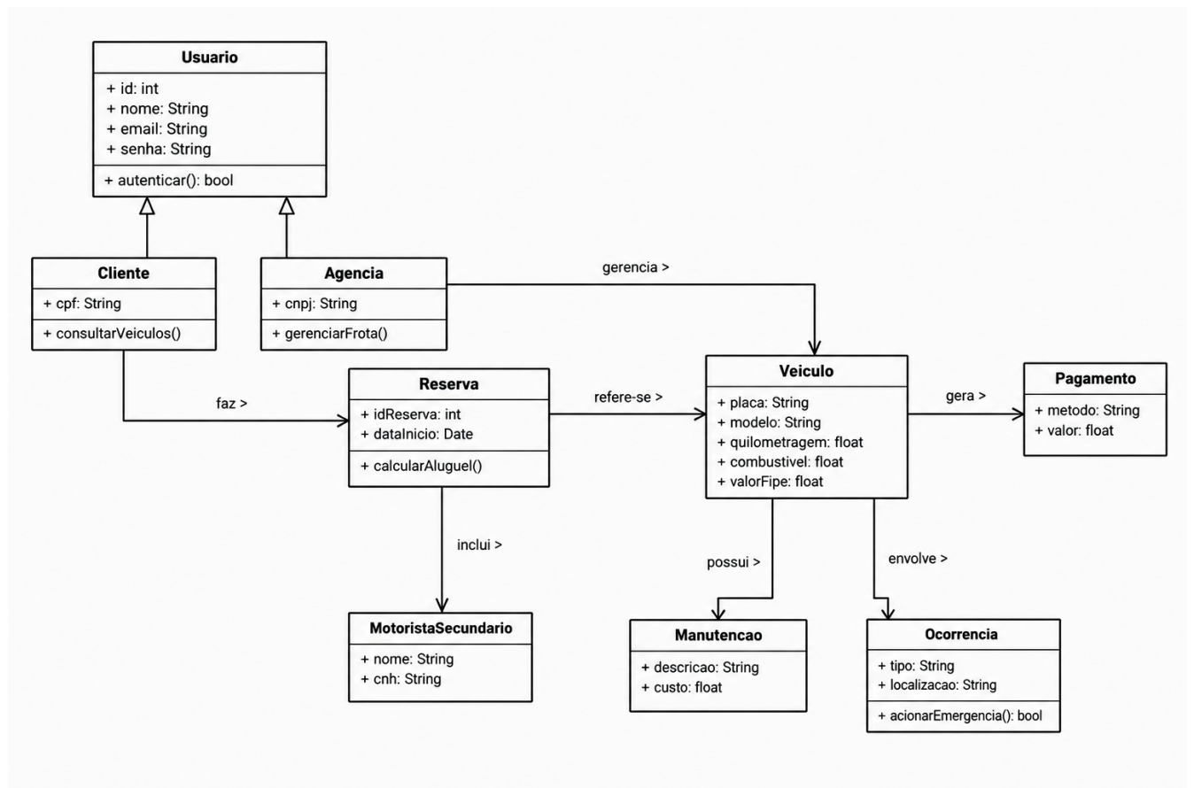
Figura 5.2: Diagrama UML
